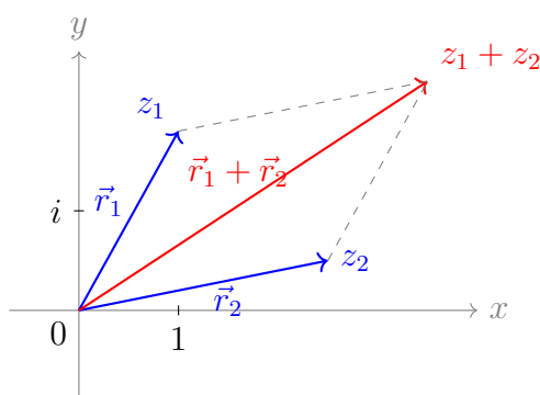
Рис. 2: Сложение комплексных чисел по правилу параллелограмма.
