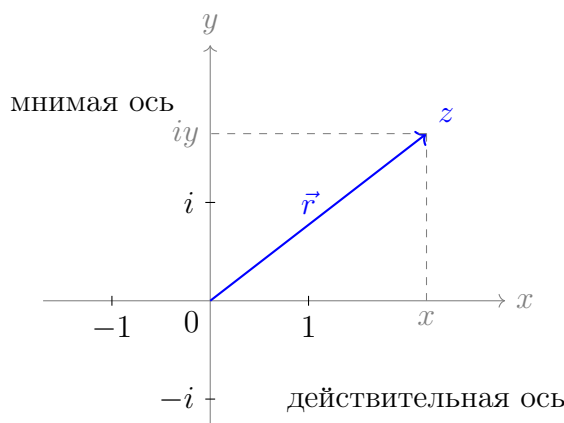
Рис. 1: Изображение комплексного числа z = x + iy точкой M(x, y) на комплексной плоскости.
