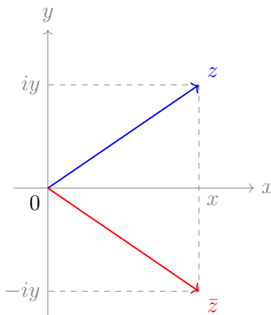
Рис. 4: Комплексно сопряжённое число \bar{z} как отражение z относительно действительной оси.
