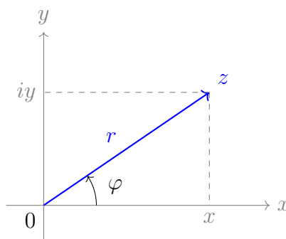
Рис. 3: Полярные координаты точки z : модуль r и аргумент \varphi .
