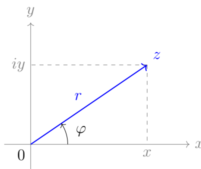
Рис. 3: Полярные координаты точки z : модуль r и аргумент \varphi .
