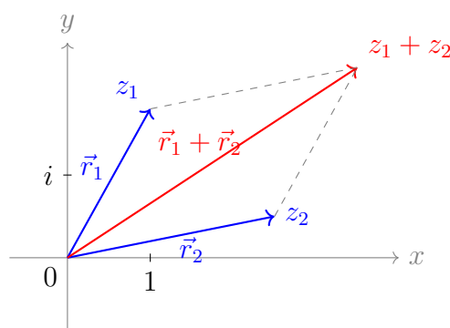
Рис. 2: Сложение комплексных чисел по правилу параллелограмма.
