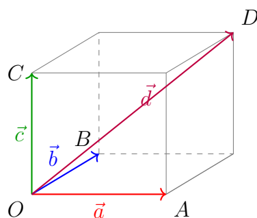
Рис. 2: \vec{d} = \alpha\vec{a} + \beta\vec{b} + \gamma\vec{c} – любой четвёртый вектор раскладывается по трём некомпланарным.
