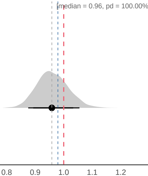
sigma_tau
