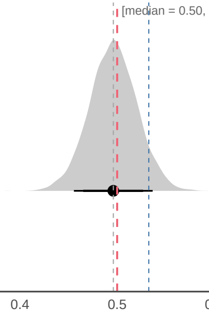
sigma_tau
