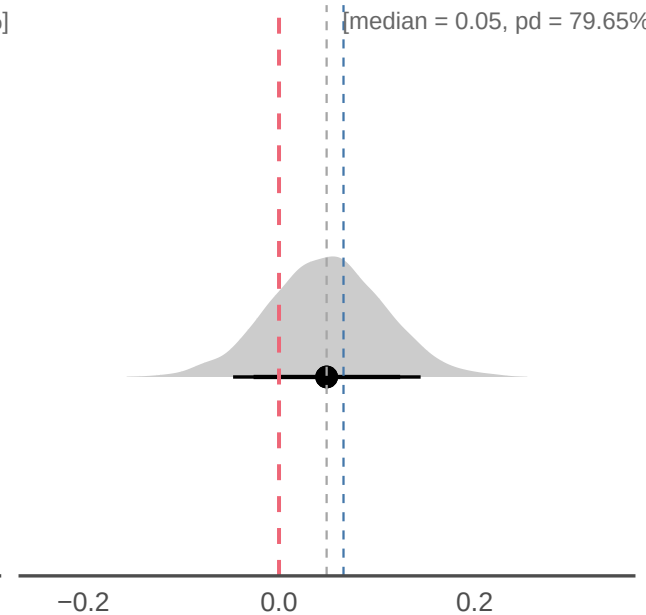
mu_rho
