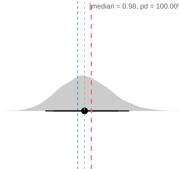
sigma_tau
