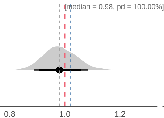
mu_rho
