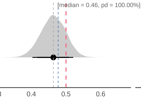
sigma_tau
