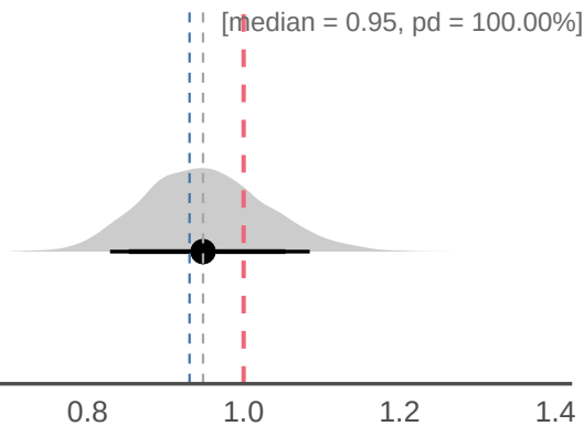
mu_rho
