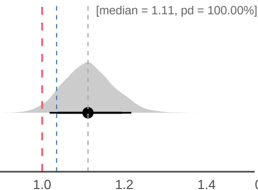
mu_rho
