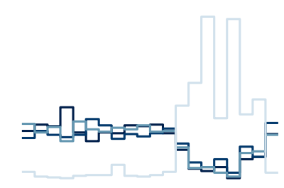
mu_tau
