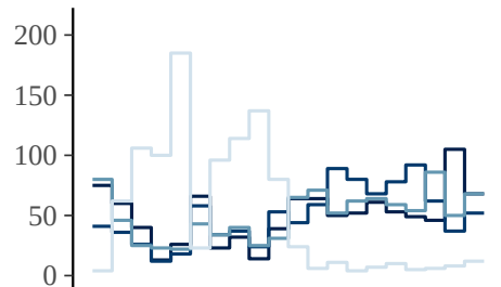
mu_log_beta
