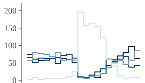
sigma_tau
