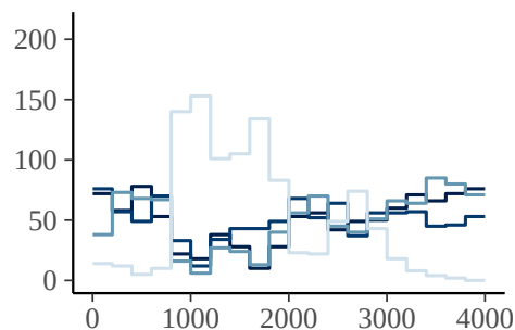
mu_rho
