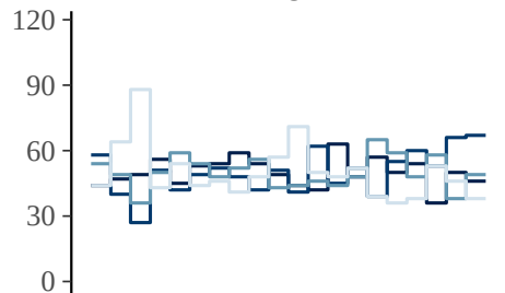
mu_log_beta
