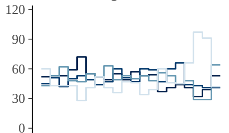
sigma_tau
