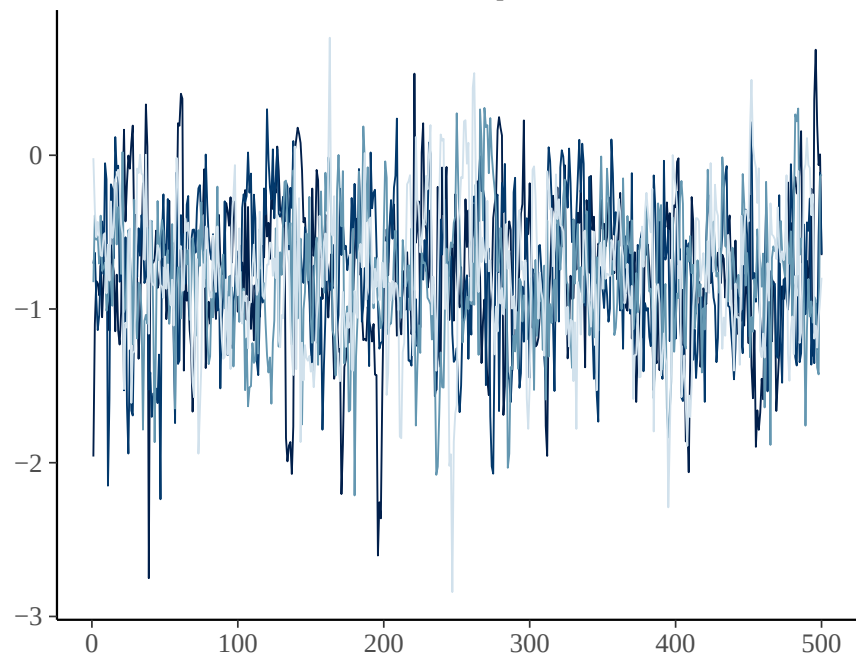
mu_beta_per
