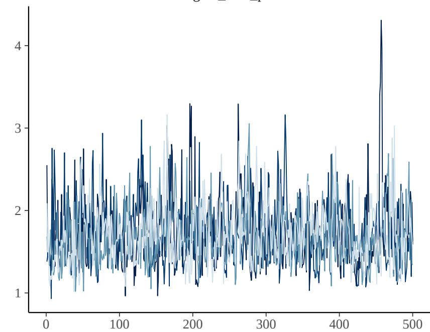
sigma_beta_per
