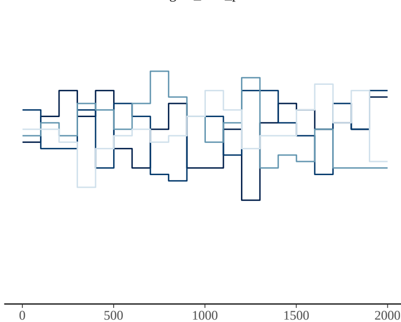
sigma_beta_per
