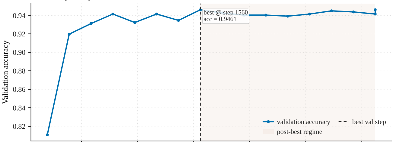
Evaluation trajectory — SST-2 · seed 42 · lr 2e-5
