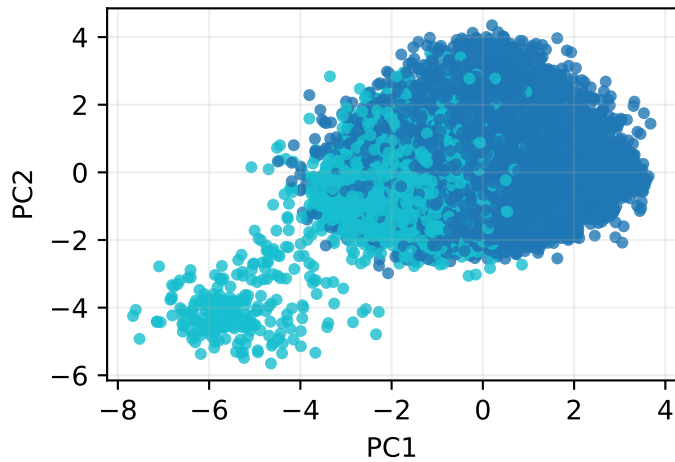
True labels
