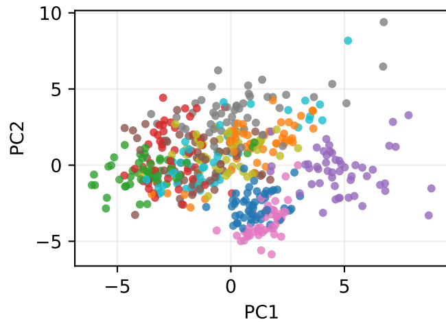
True labels
