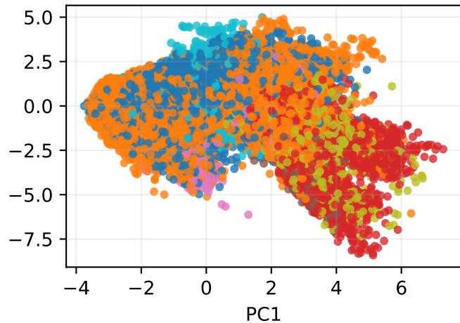
True labels
