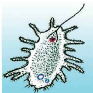
Расми 40. Мастигоамёба
