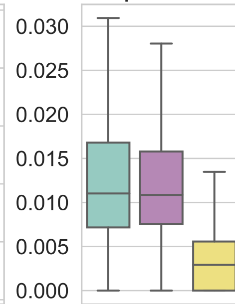
FKGL
