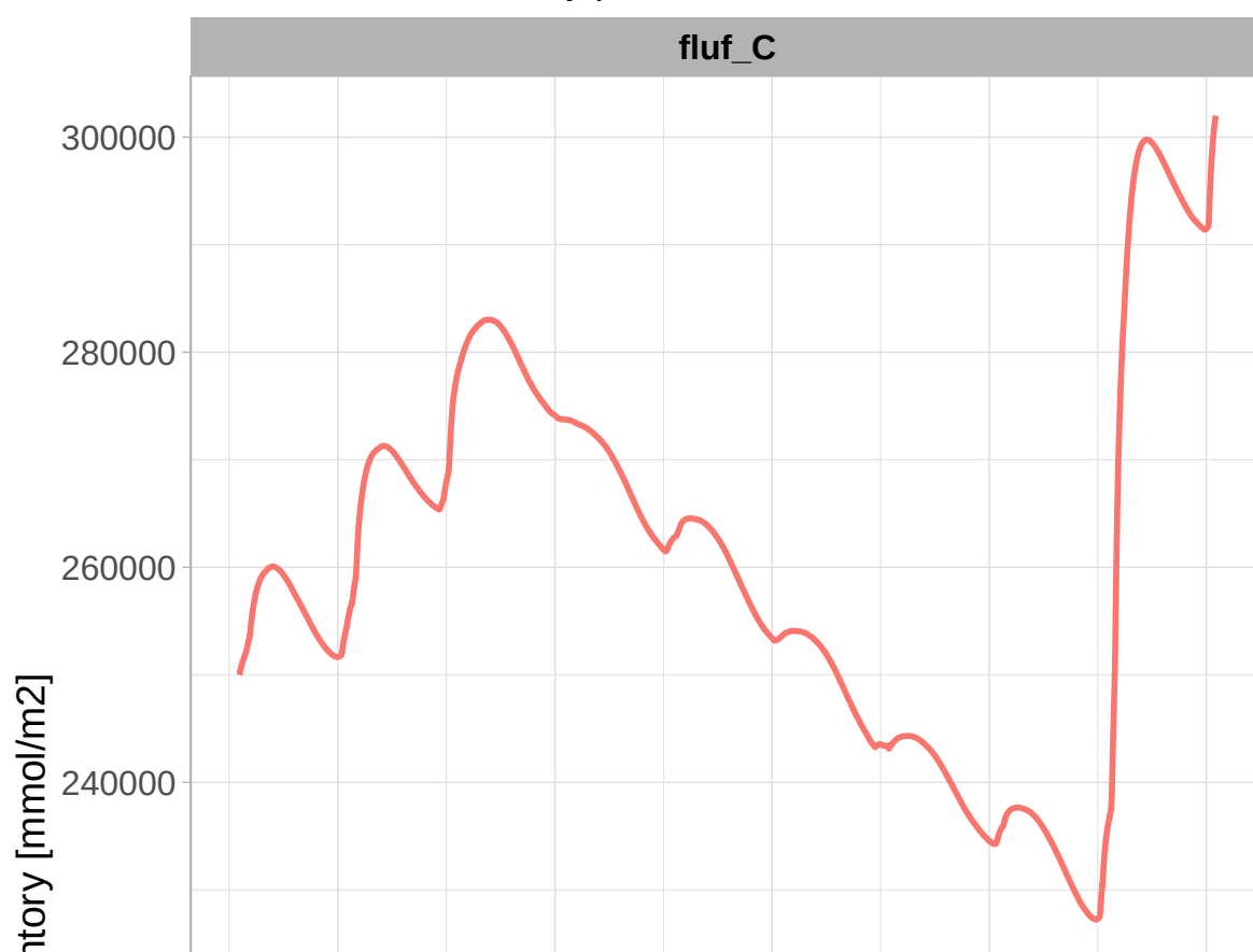
Mean sediment inventory per bottom area
