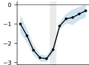
(e) v850, BD ( \text{m s}^{-1} )
