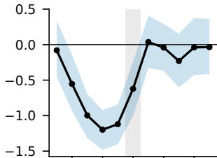
(e) v850, BD ( \text{m s}^{-1} )
