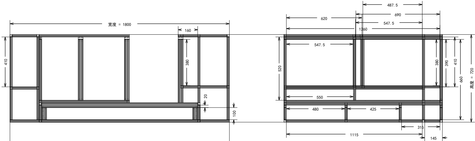
前视图
