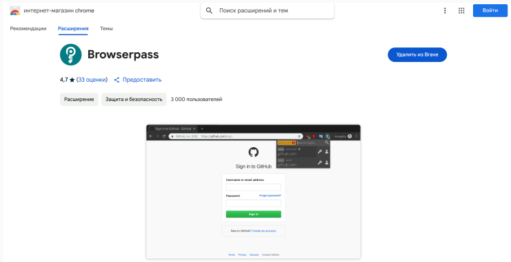
Рис. 8: Скачивание расширения
