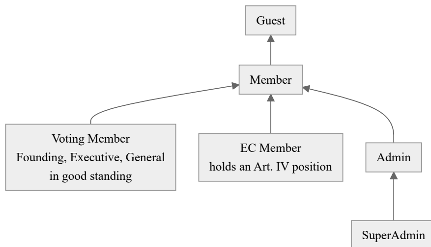
Fig. 3.7. Actor generalisation hierarchy
