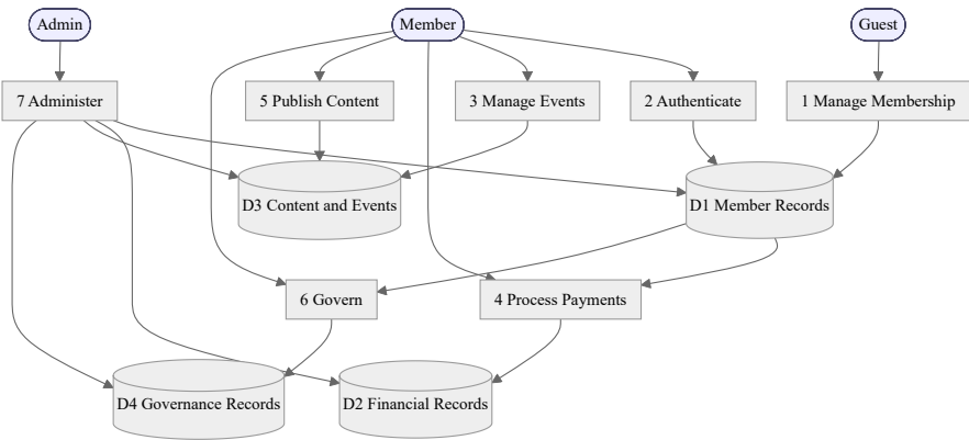
Fig. 5.2. DFD Level 1
