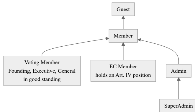
Fig. 3.7. Actor generalisation hierarchy
