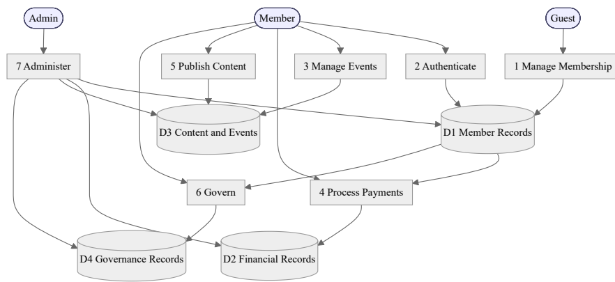
Fig. 5.2. DFD Level 1
