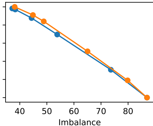
Noisy Karloff
