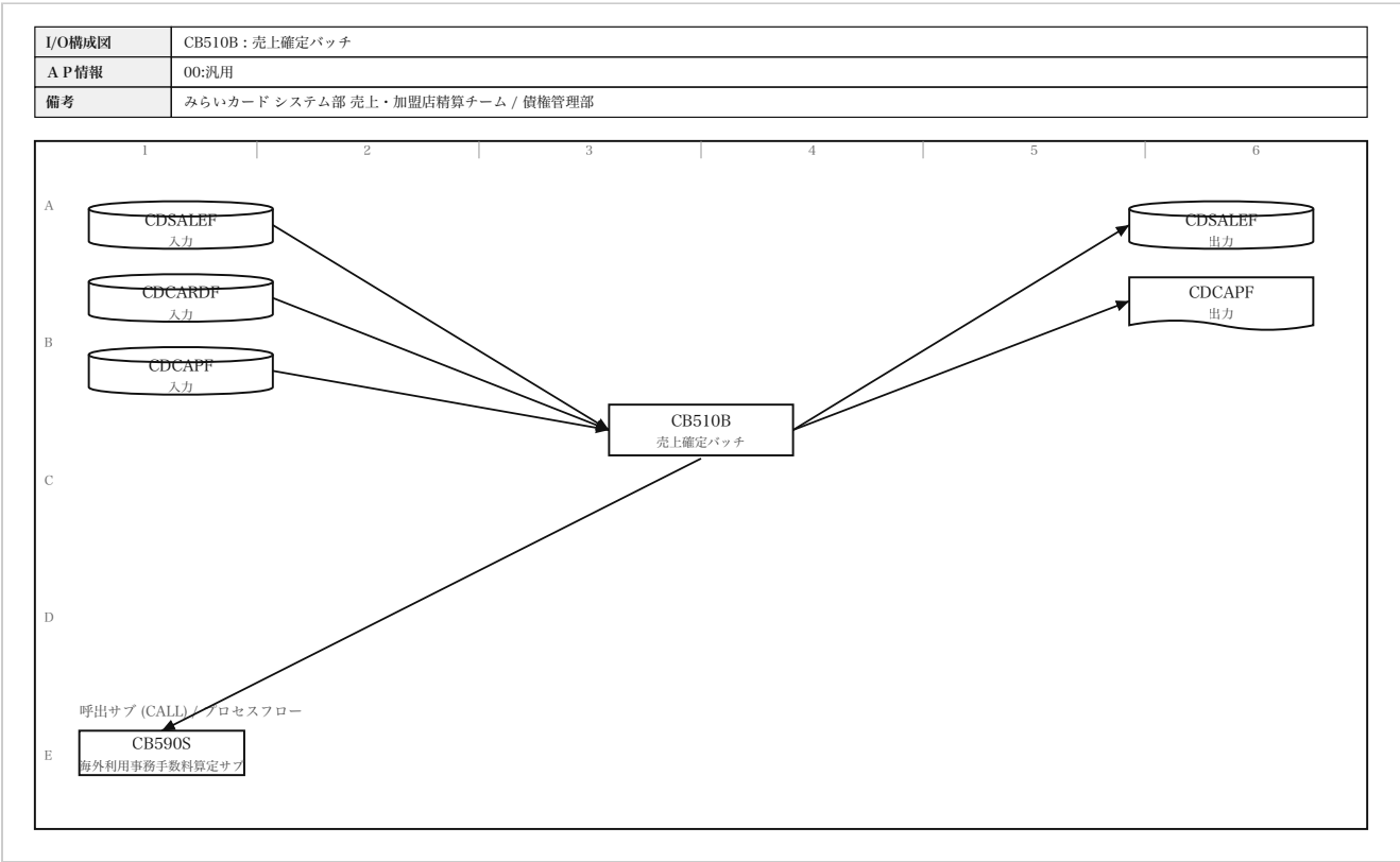
図1 入出力構成および呼出サブの実行順序。
