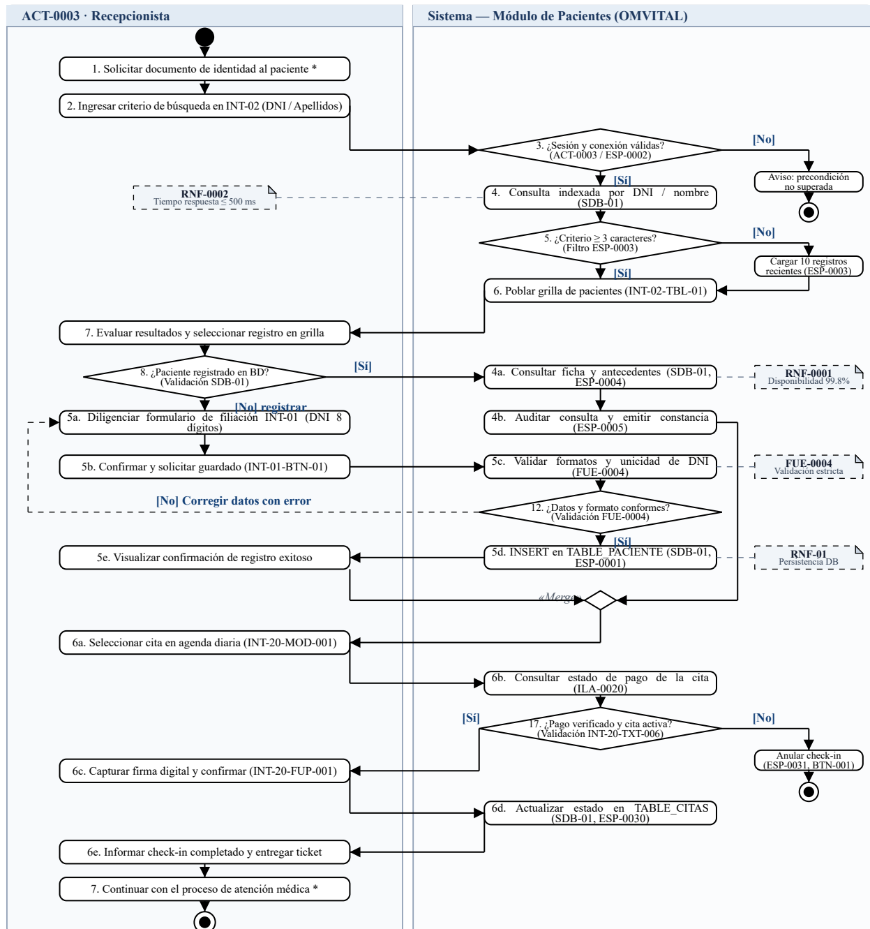
Figura 2: DIA-CMP-0001 : Diagrama de comportamiento de Nivel 2 (UML 2.5): descomposición detallada de «2. Identificar paciente» (ESP-0003), «4. Consultar / cargar ficha del paciente» (ESP-0004 / ESP-0005), «5. Registrar nuevo paciente» (ESP-0001 / ESP-0002 / FUE-0004) y «6. Iniciar check-in en agenda diaria» (ESP-0030 / ESP-0031), con carriles de proceso Recepcionista/Sistema, guardas [Si]/[No] y bucle de validación FUE-0004; conserva la decisión y el nodo de fusión del Nivel 1.
