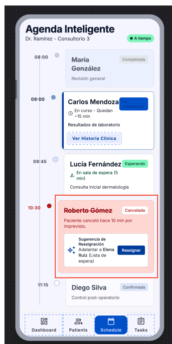
Figura 4: Mockup de la aplicación Medifácil la parte de Agenda
