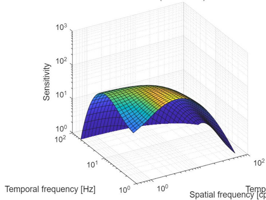
Achromatic (Luminance)
