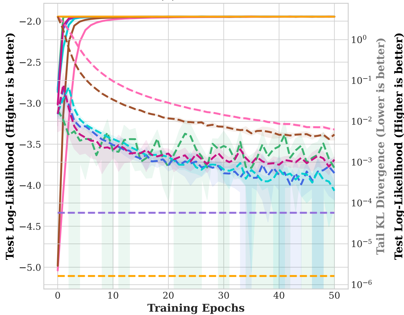
(a) Poisson
