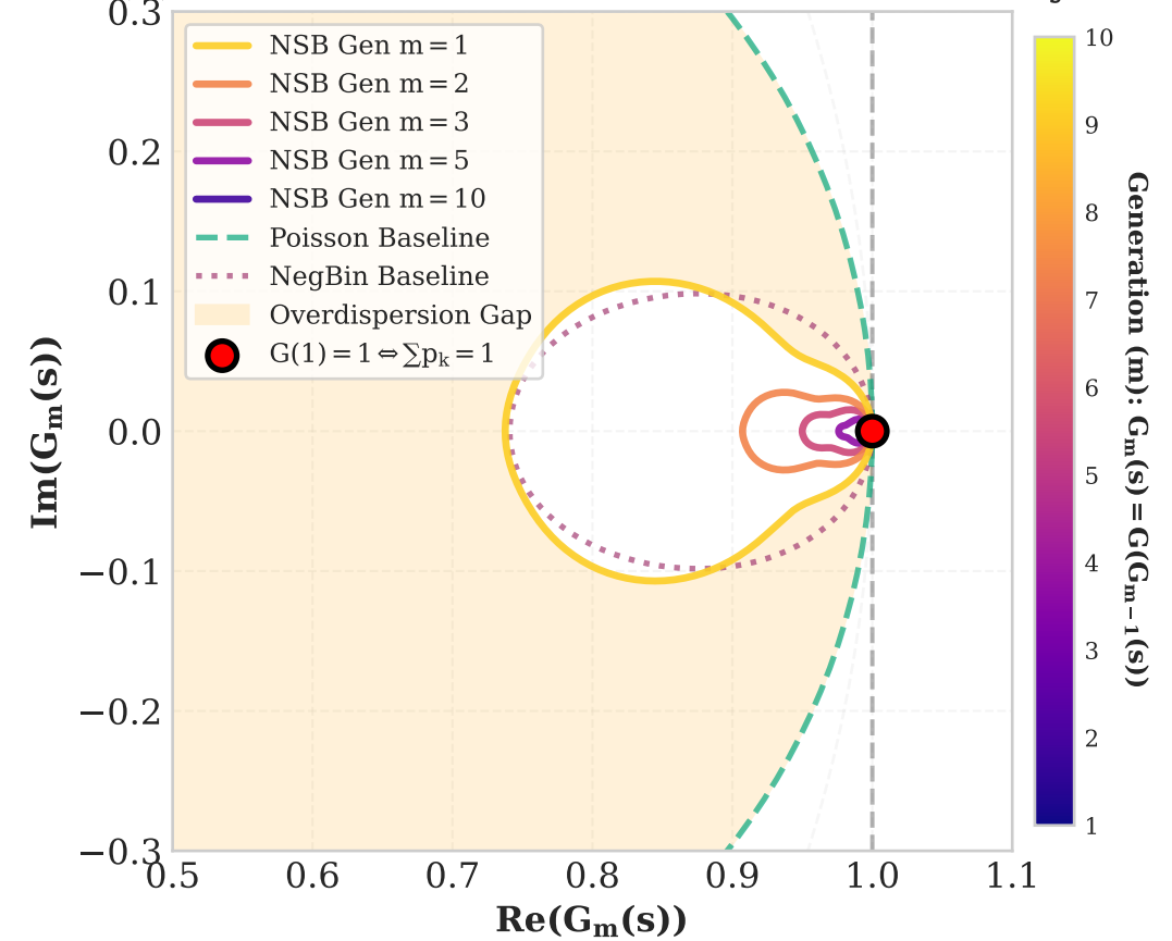
(d) Generational Loss of Forensic Memory
