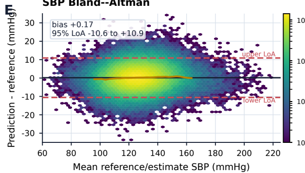
SBP Bland--Altman
