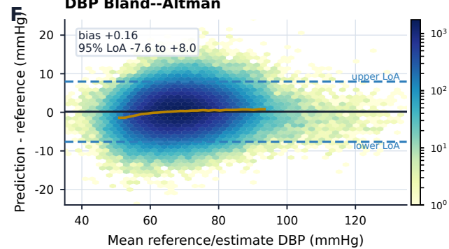
DBP Bland--Altman
