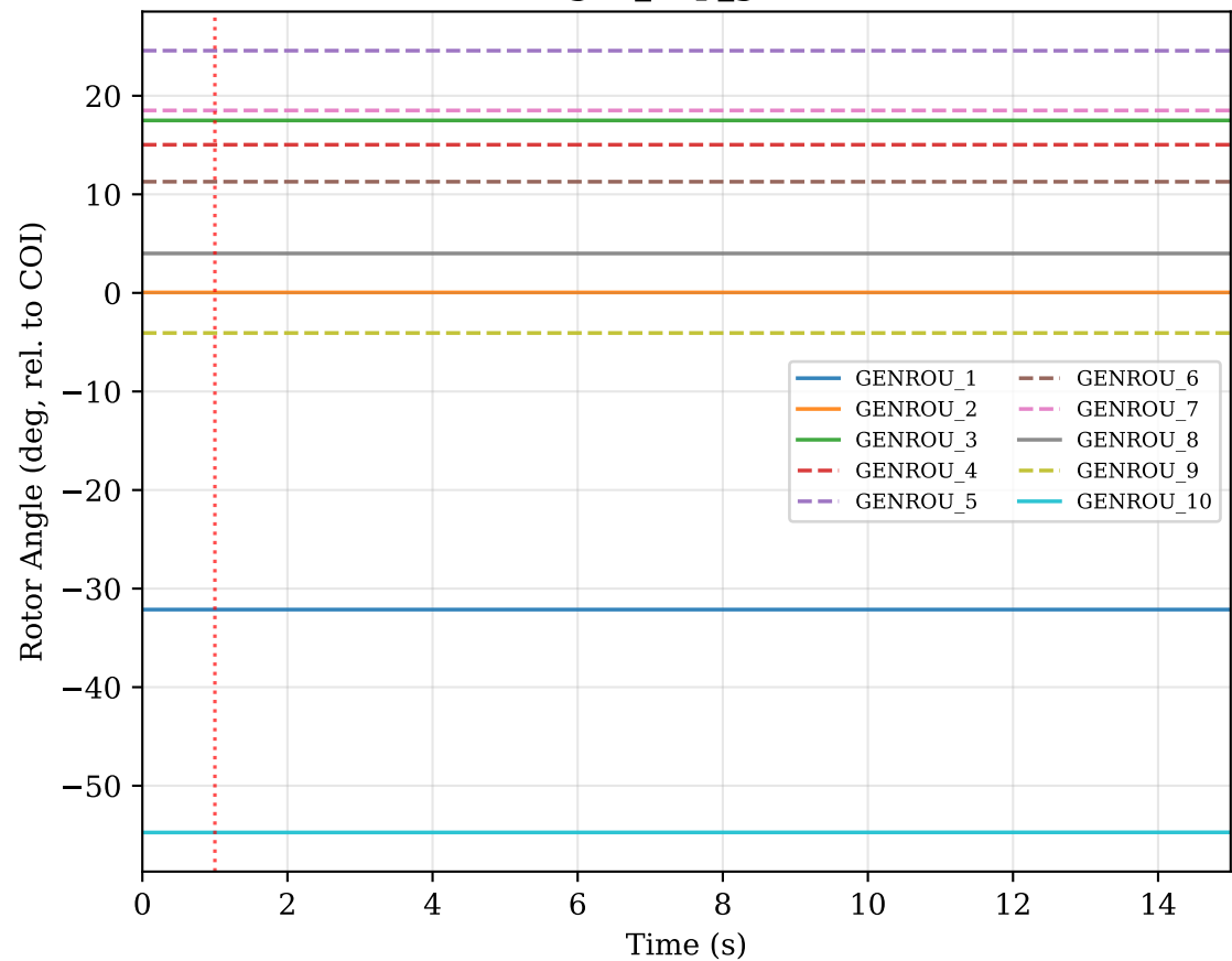
(b) Stable: gen_trip_g4 (sev=0.220)
