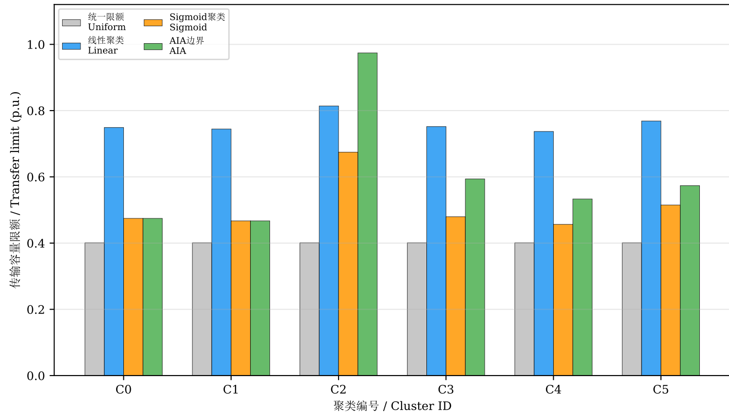
图7 分场景传输容量限额对比 Fig. 7 Per-scenario transfer limit comparison
