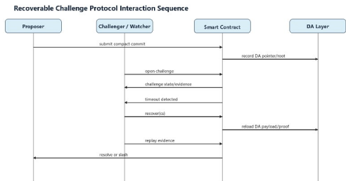
图 2 RCP 协议交互时序
