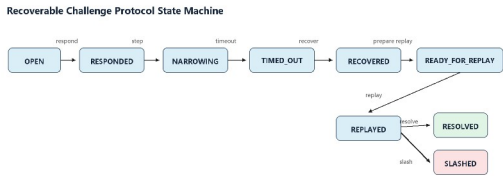
图 3 可恢复挑战协议状态机
