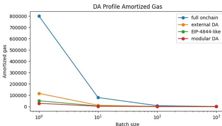
图 4 不同数据可用性配置下的摊销 gas 用量趋势
