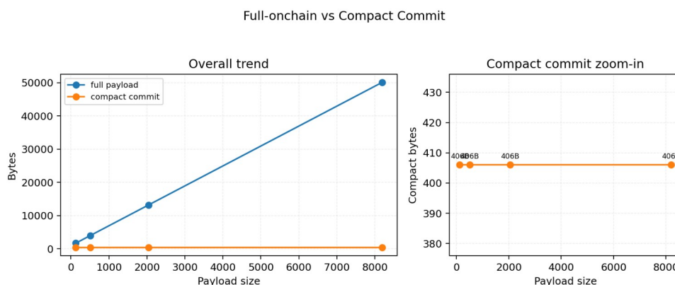
图 3 完整负载与紧凑提交的字节规模对比
