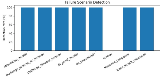
图 6 失败场景检测与仲裁结果
