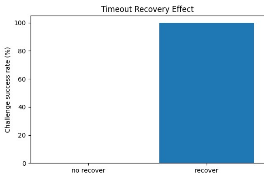
图 2 恢复对超时场景挑战完成率的影响
