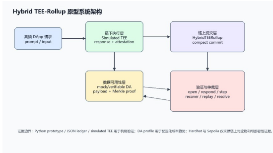
图 1 可恢复挑战驱动的 Hybrid TEE-Rollup 原型架构
