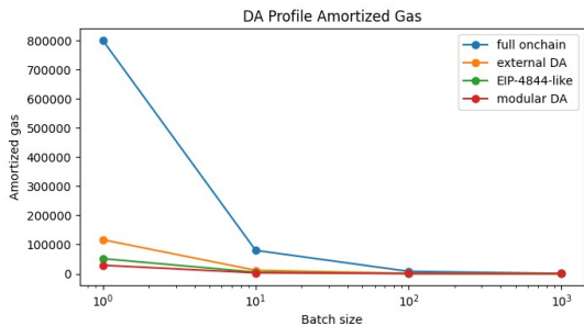
图 5 不同 DA profile 下的摊销 gas 趋势
