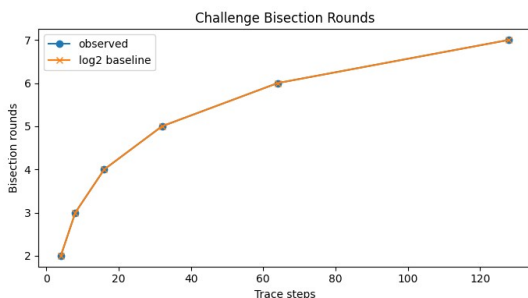
图 3 二分挑战轮次与 trace steps 的关系
