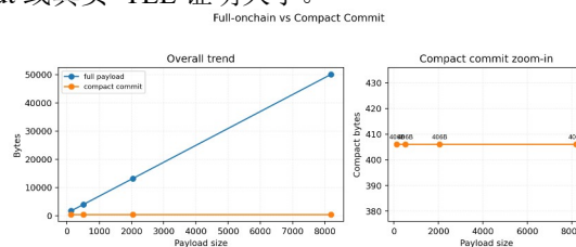
图 4 full payload 与 compact commit 的字节规模对比
