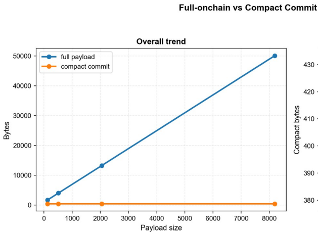
图 7 full payload 与 compact commit 的字节规模对比
