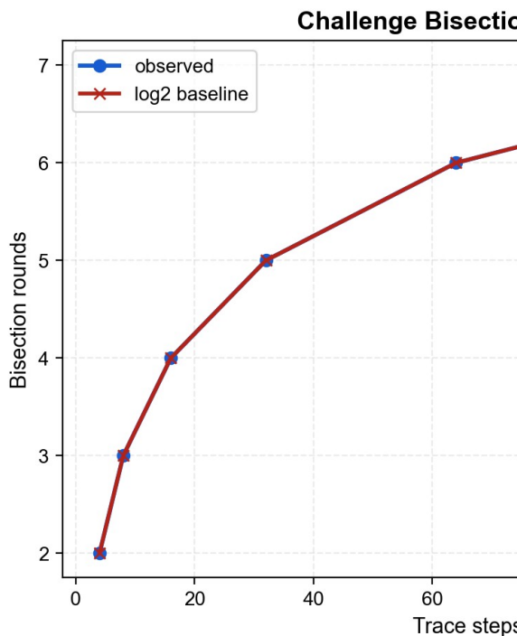
图 6 二分挑战轮次与 trace steps 的关系 7.4 RQ3: 紧凑提交是否提供稳定证据锚点
