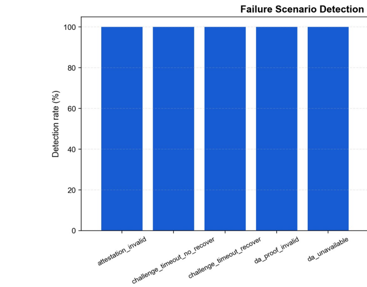
图 9 失败场景检测与仲裁结果
