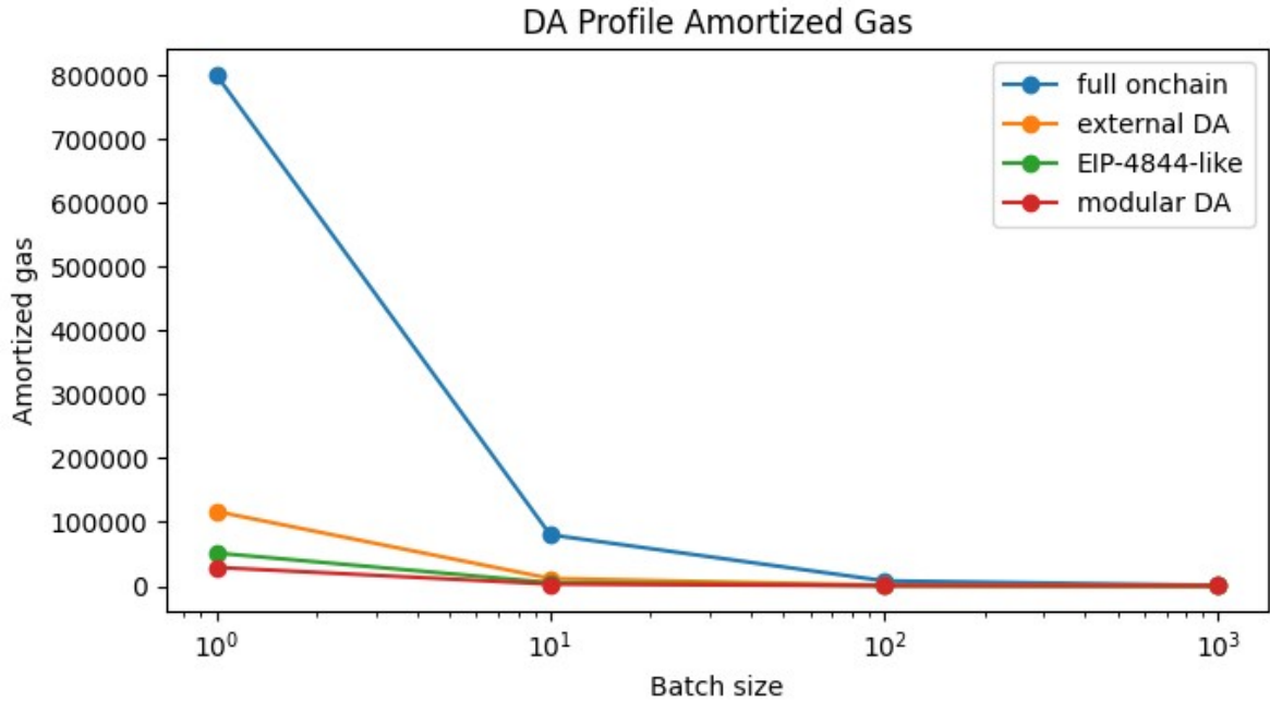
图 4 不同 DA profile 下的摊销 gas 趋势
