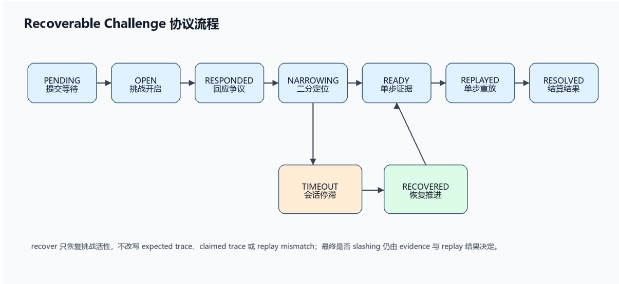
图 2 Recoverable Challenge 协议流程
