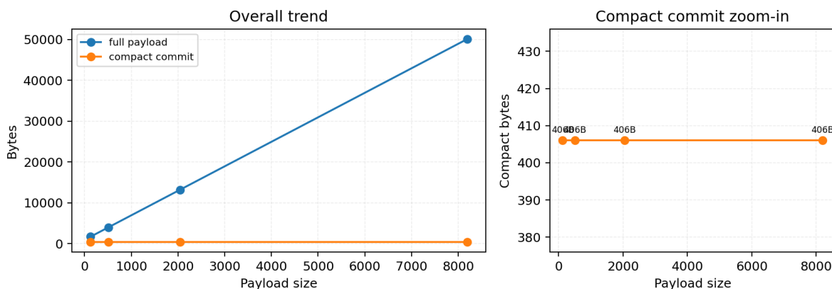
图 3 full payload 与 compact commit 的字节规模对比
