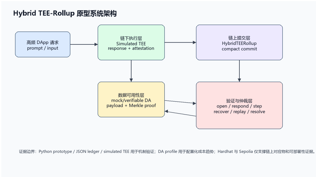
图 1 Hybrid TEE-Rollup 原型系统架构
