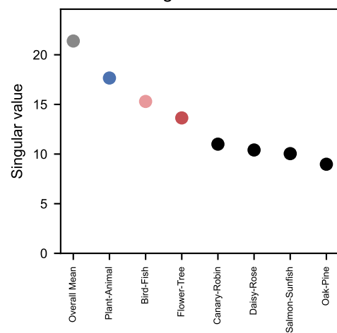
Singular values
