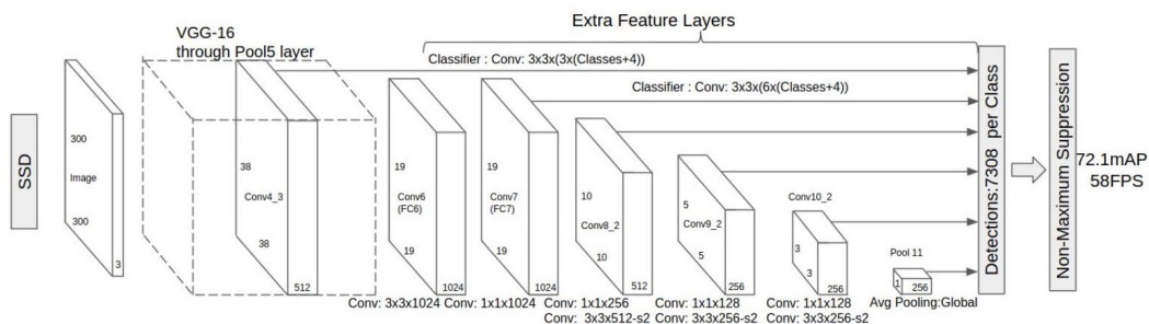
图 1-1 SSD 模型结构
