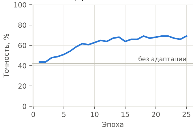
(b) Точность на dev
