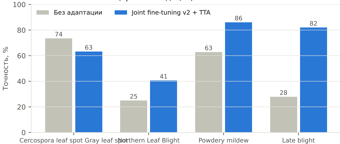
Точность по классам (кросс-валидация)
