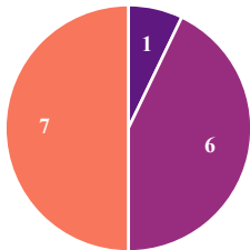
LIBERO (n = 14)
