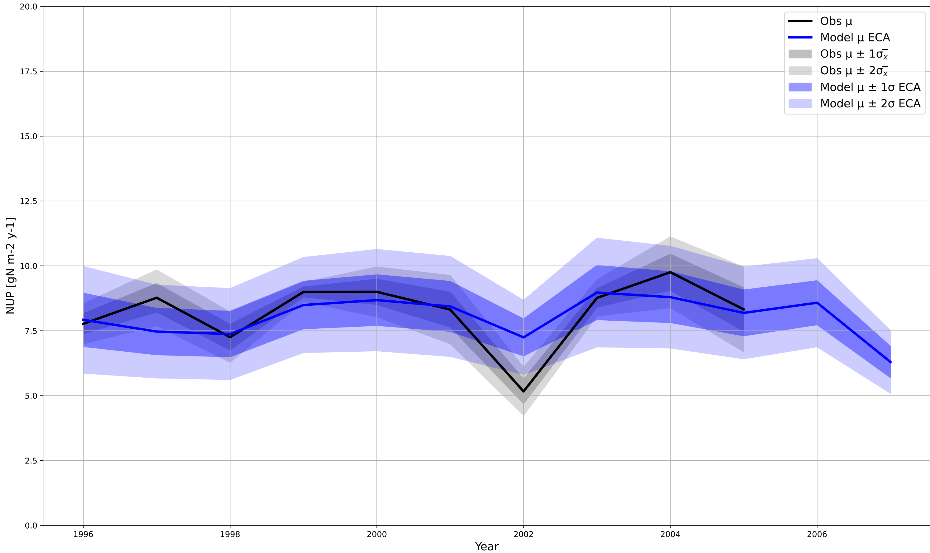
NUP Models and Obs DUKE - AMB - ECA 3
