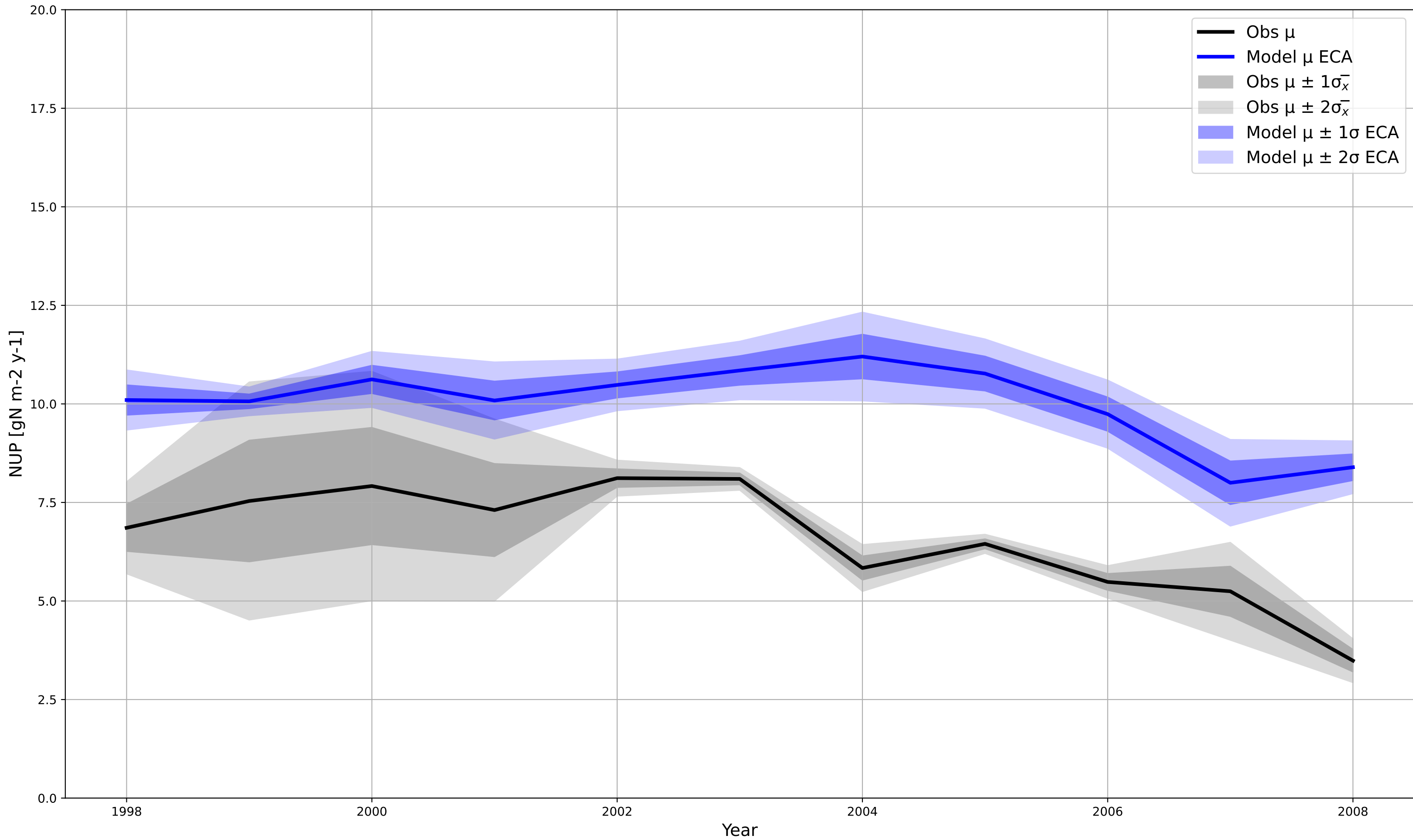
NUP Models and Obs ORNL - AMB - ECA 3
