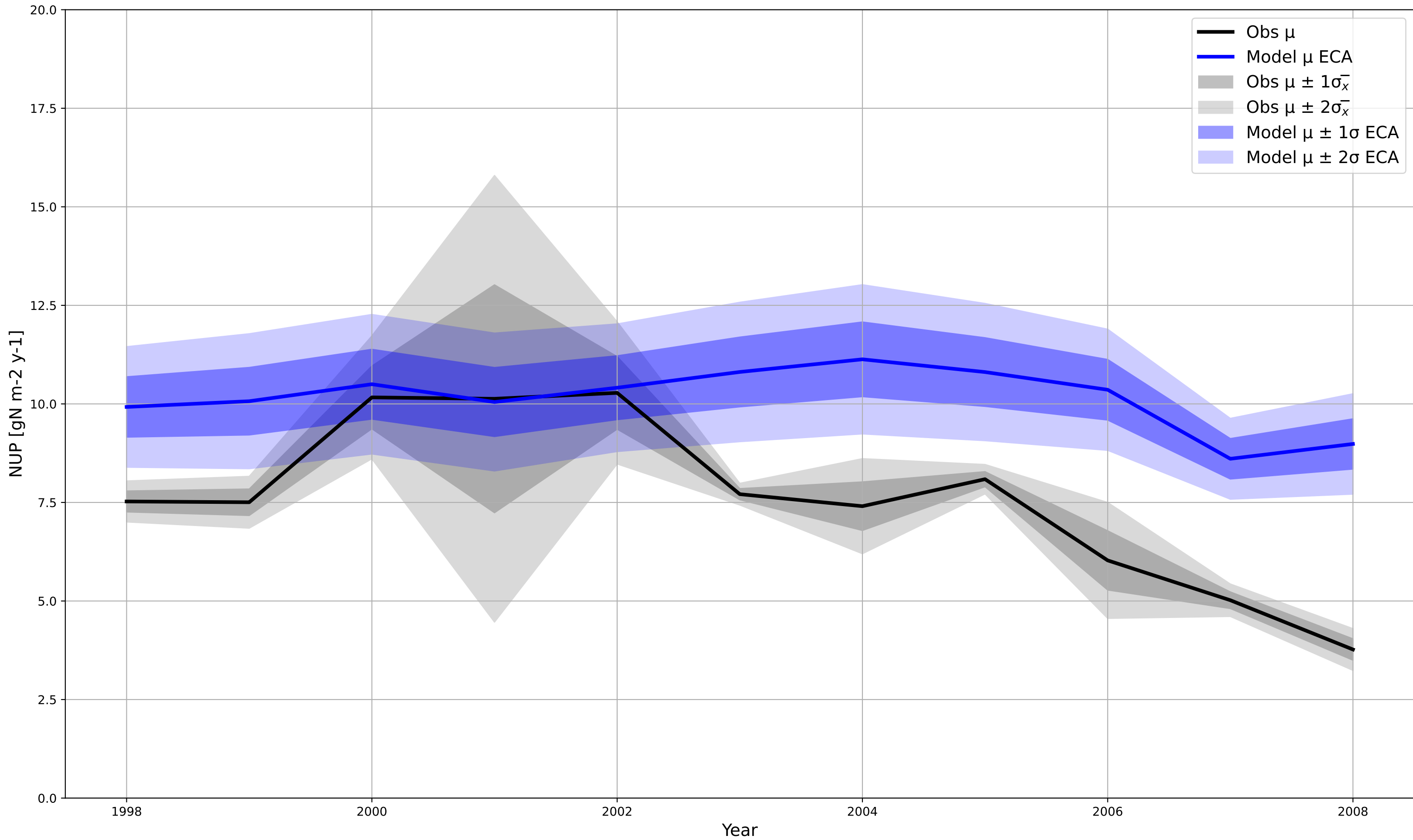
NUP Models and Obs ORNL - ELE - ECA 2
