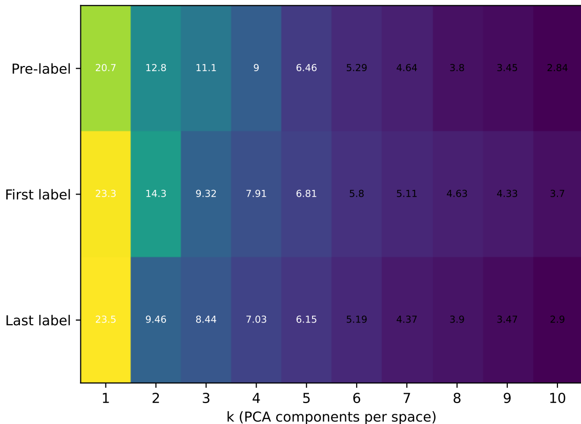
Train-task MSE
