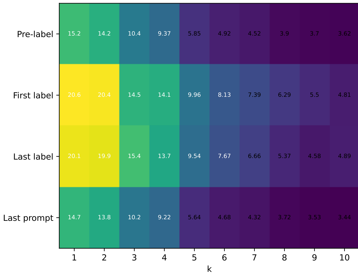
Train-task MSE
