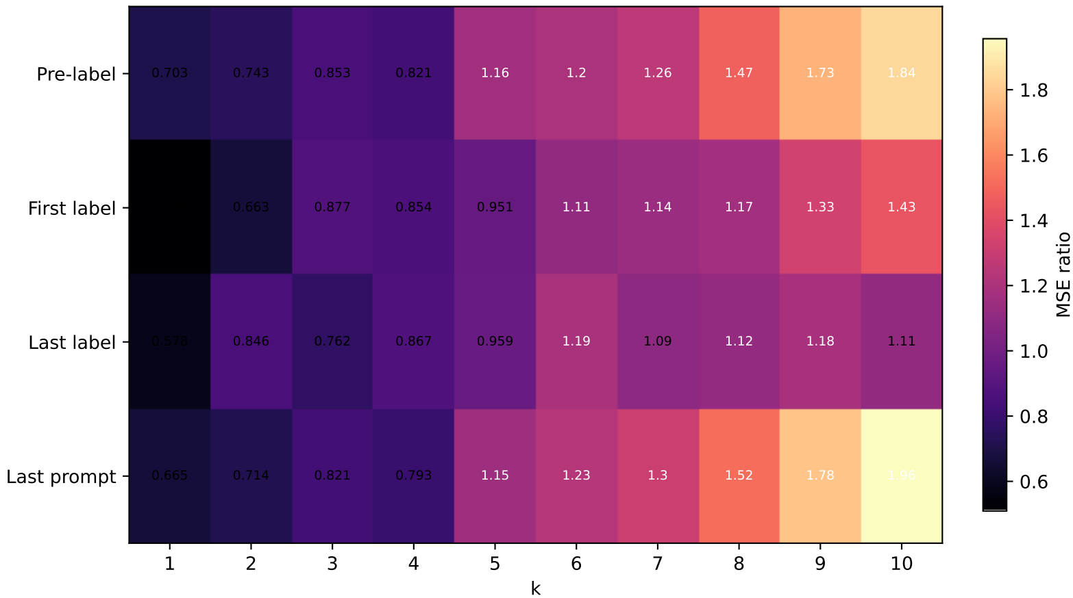
Held-out test MSE / train MSE
