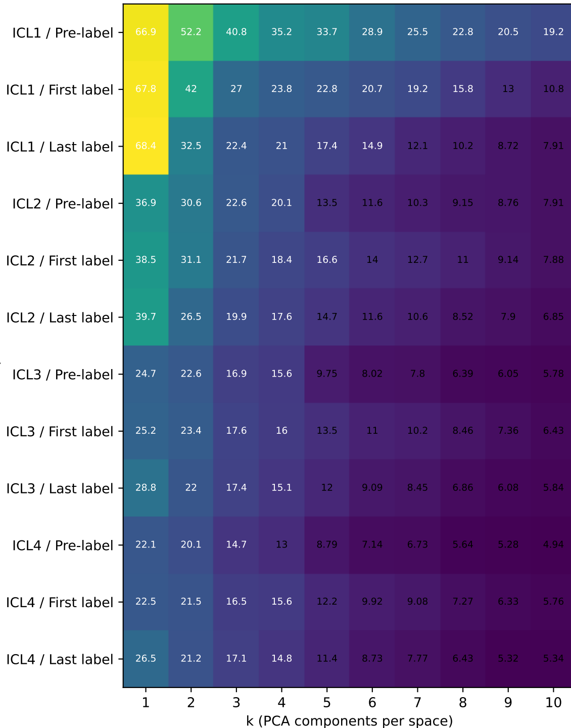
Train-task MSE
